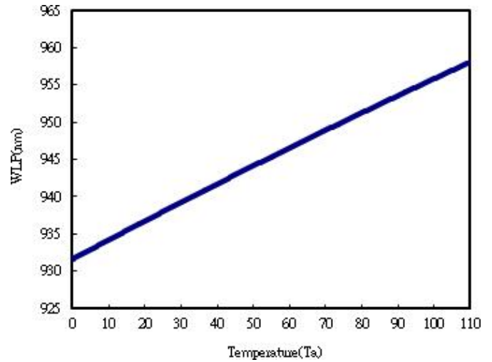
Fig.10 The WLF shift vs Ta(°C)
